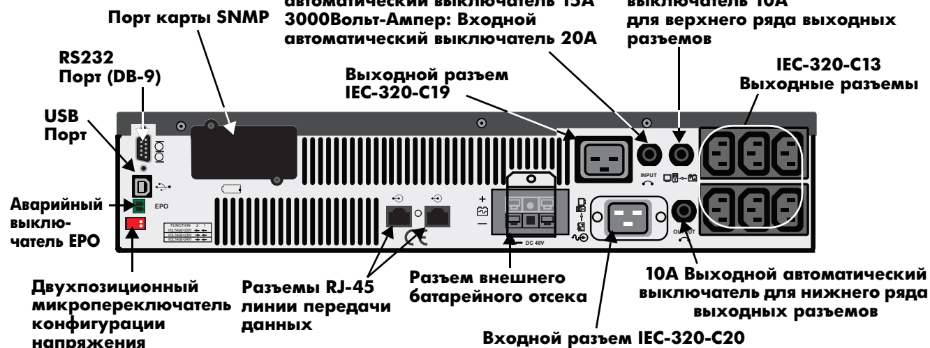
Рисунок 3 2200 и 3000VA—вид сзади
