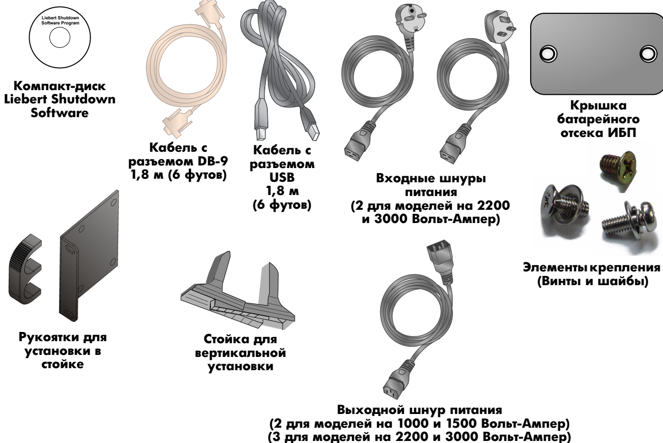
Рисунок 4 Дополнительное оборудование
